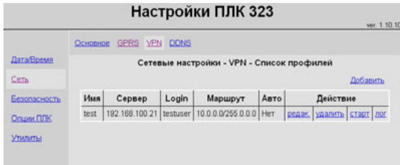
Рисунок Г.9 – Окно настройки VPN
