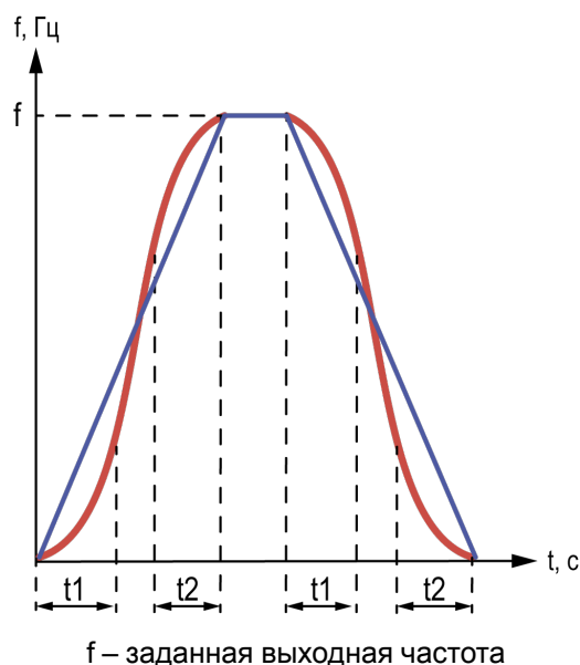
Рисунок 2.2 – S-образная кривая разгона и торможения A
